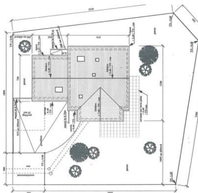
Exemple de plan de masse
