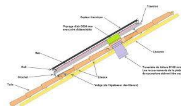
Exemple de plan en coupe
